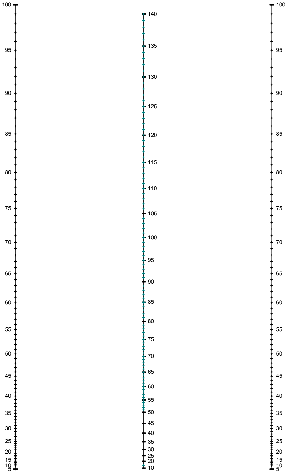
שתי טעויות דגימה של X_1 Two Sampling Errors For X_1
