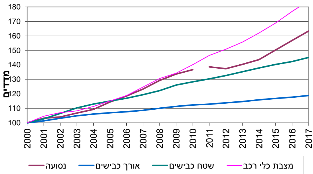
תרשים 1 - נסועה שנתית, מצבת כלי הרכב, שטח הכבישים ואורכם 2017-2000 בסיס: 2000=100
